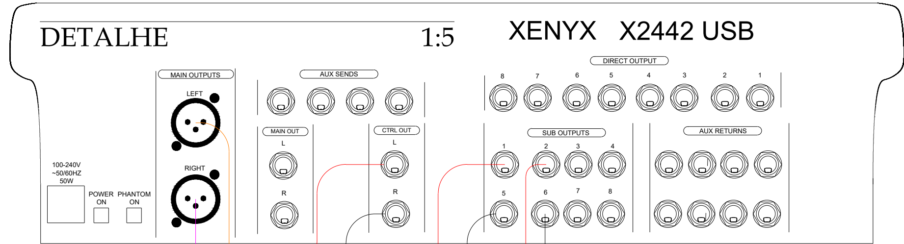
DETALHE PARTE TRÁS DA BEHRINGER XENYX X2442 USB
